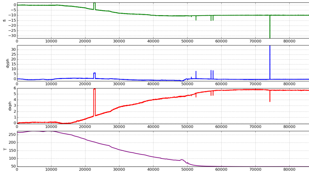
Рисунок 4.2 –Зависимость от времени в секундах критериальных параметров реальных перемещений ПГ № 2
